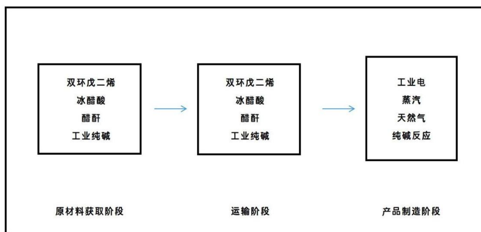
图2-1 产品碳足迹评价系统边界
